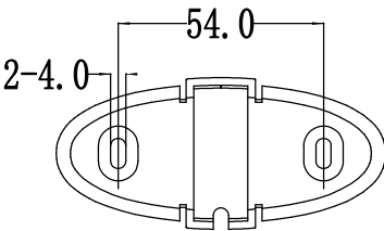
风光雨传感器螺钉孔尺寸和安装孔 间距尺寸:
